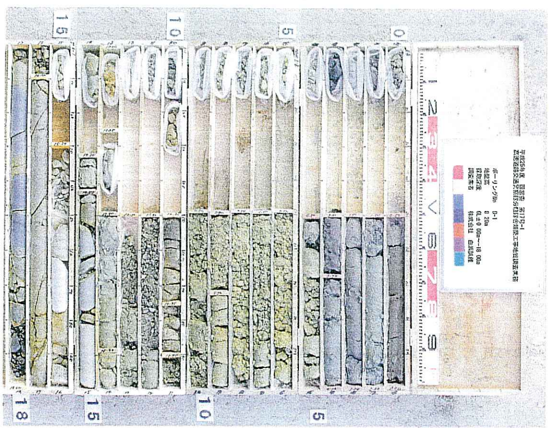
ボーリングコア写真 B-1 (GL ± 0.00m ~ -18.00m)
